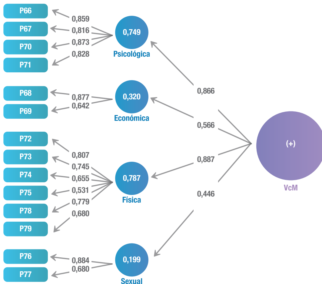
Figura 1. Estructura factorial de segundo orden de la escala de violencia contra las mujeres en relaciones de pareja usando SEM-PLS.
